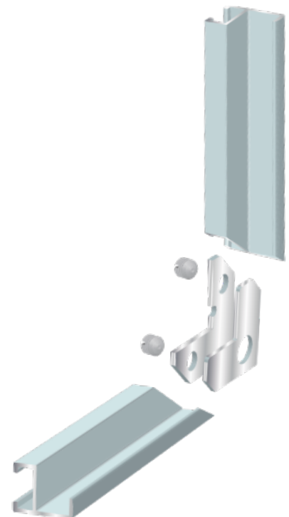
Taulukehyksen kulmaliitospala sis. ripustuskoukut, jouset
